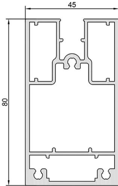
23-7113 KAPI PROFİLİ Ağırlık / Weight = 2,094 kg/m ÖLÇEK : 1/1
