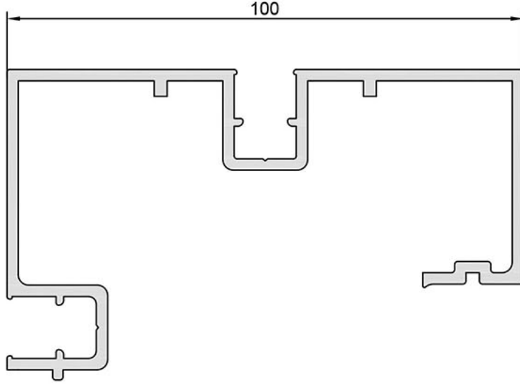
23-7189 100 mm Panel PROFİL Ağırlık / Weight = 1,787 kg/m
