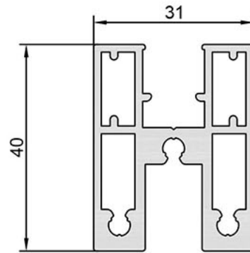
23-7140 * TRABZAN PROFİLİ Ağırlık / Weight = 1,223 kg/m
